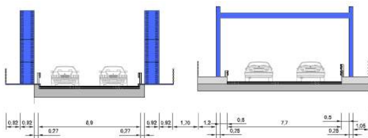
Secciones de los puentes sobre el río Gállego en situación actual. Elaboración propia.
